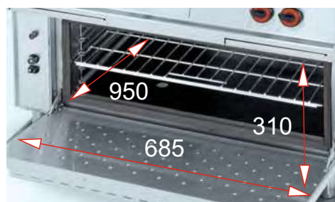
Medidas horno pasante
